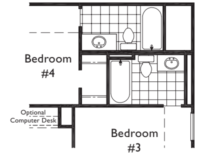
2 Full Baths Option in lieu of Jack & Jill Bath 1300-02
